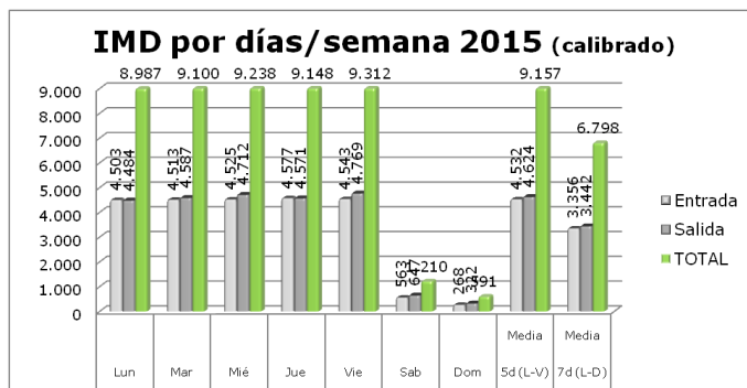
Gráfico 7. I.M.D. por días de semana y medias Centro de Transportes de Coslada4.
