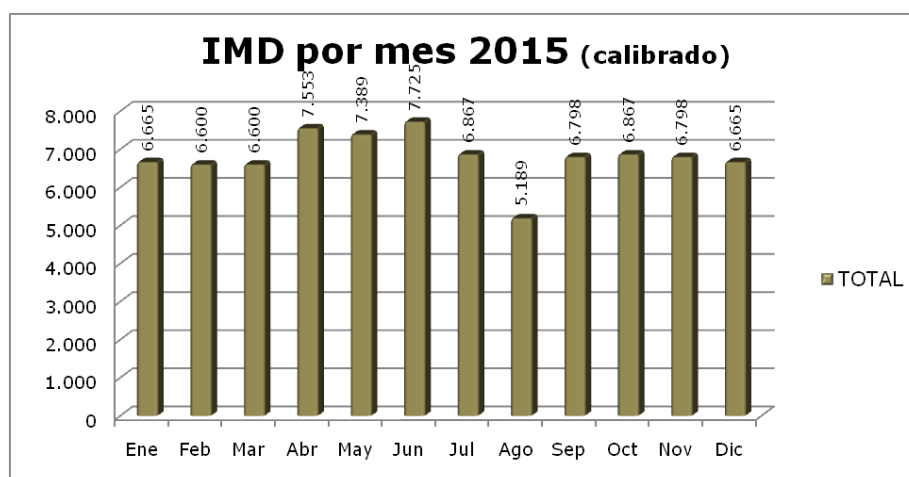
Gráfico 8. I.M.D. por meses del años
