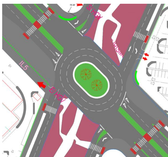
Imagen 35. Descripción solución glorieta adoptada para la intersección entre Calle A y Vía Pecuaria.
