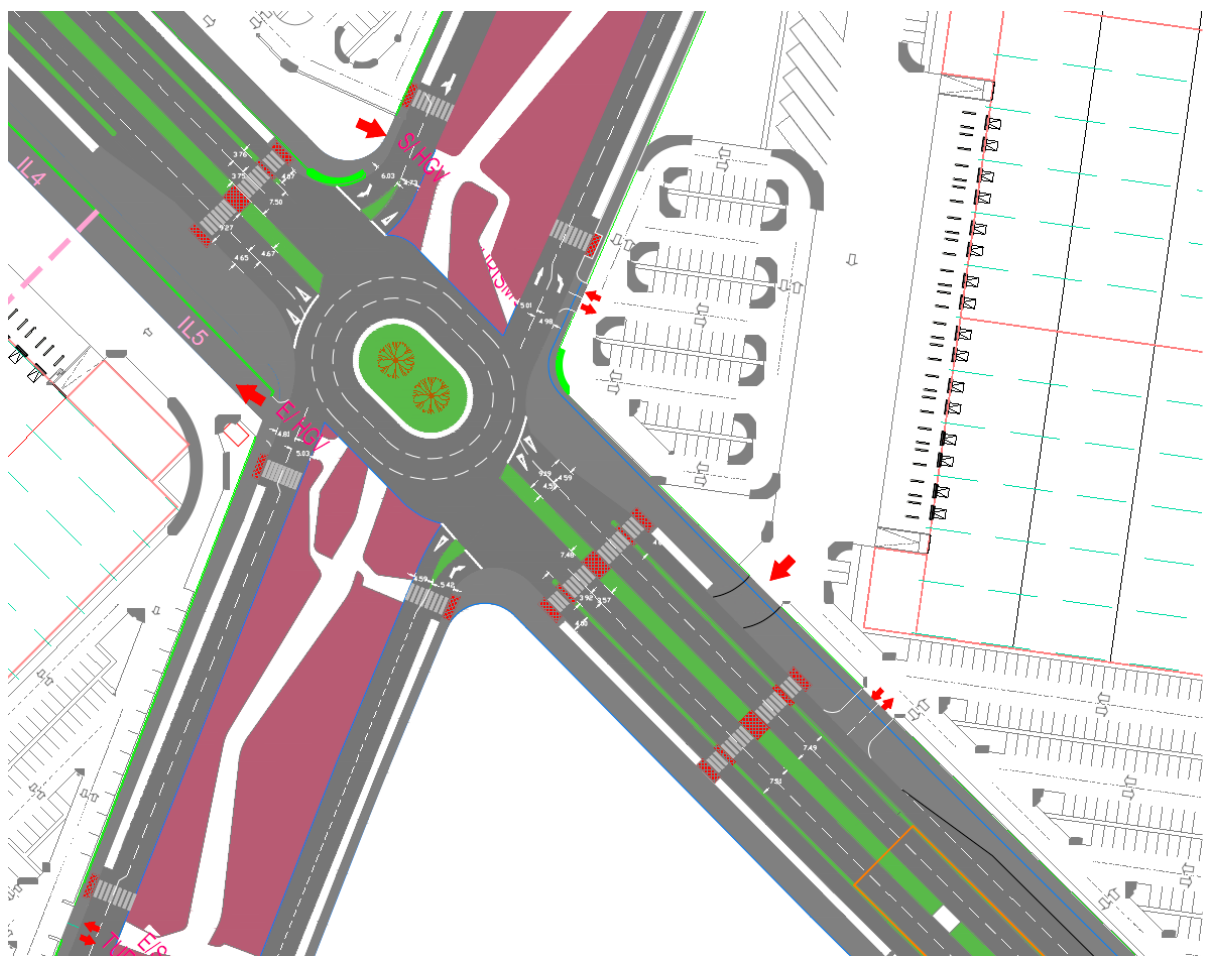
Imagen 38. Esquema de las dimensiones de la vía de servicio y carriles centrales de la Calle A.
