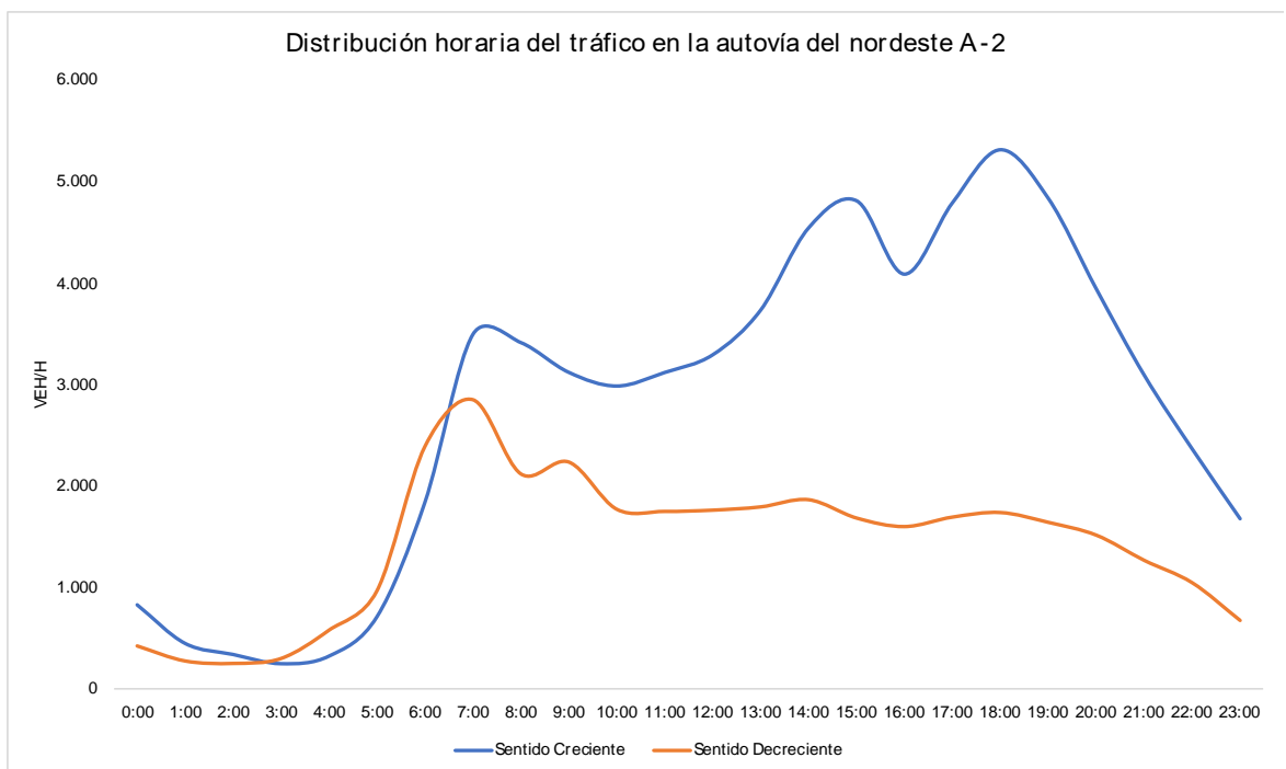
Gráfico 2. Distribución horaria del tráfico en la autovía del nordeste (A-2) durante el día laborable medio anual.
