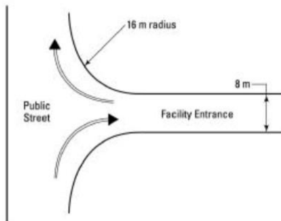
Imagen 33. Detalle de acceso en "Y".
