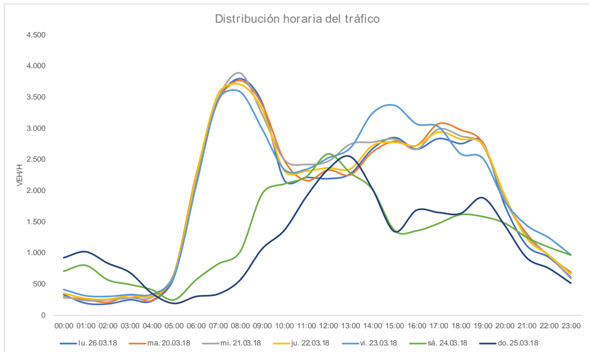
Gráfico 5. Distribución horaria del tráfico en carretera M-206.
