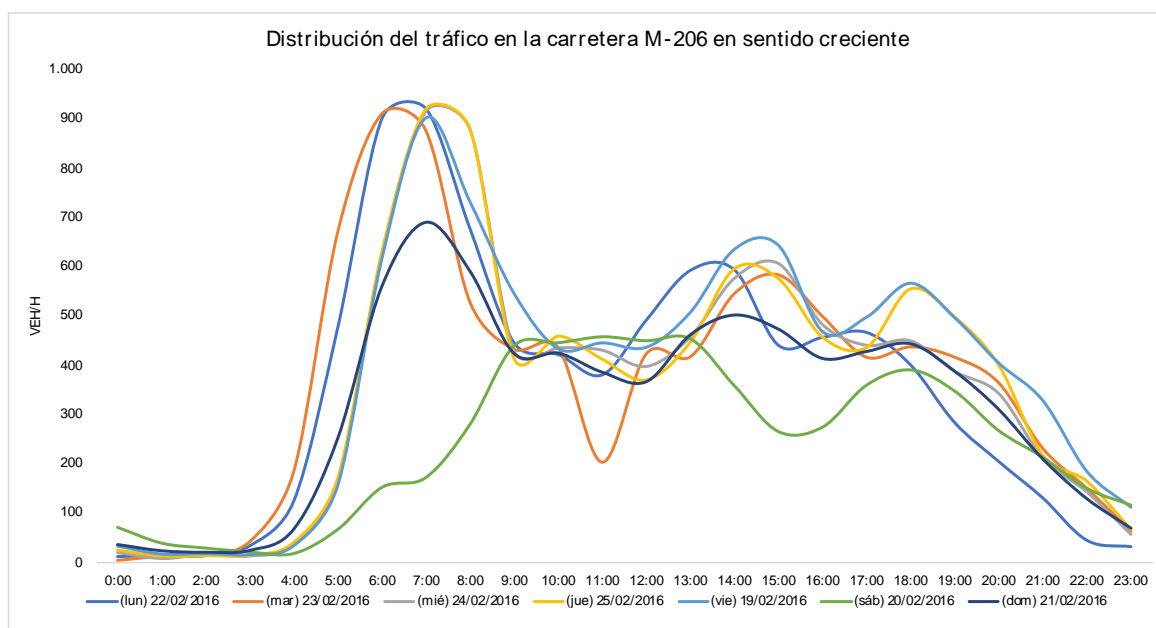
Gráfico 3. Distribución horaria del tráfico en la carreteras M-206 en sentido creciente.
