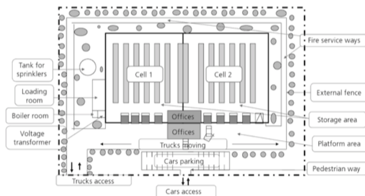
Imagen 32. Ejemplo de ordenación de centro logístico con separación de flujos de tráfico pesado y vehículos ligeros.
