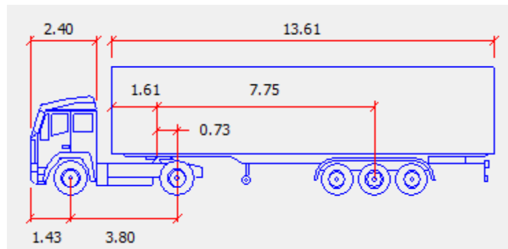
Imagen 31. Dimensiones del vehículo empleado en la simulación.
