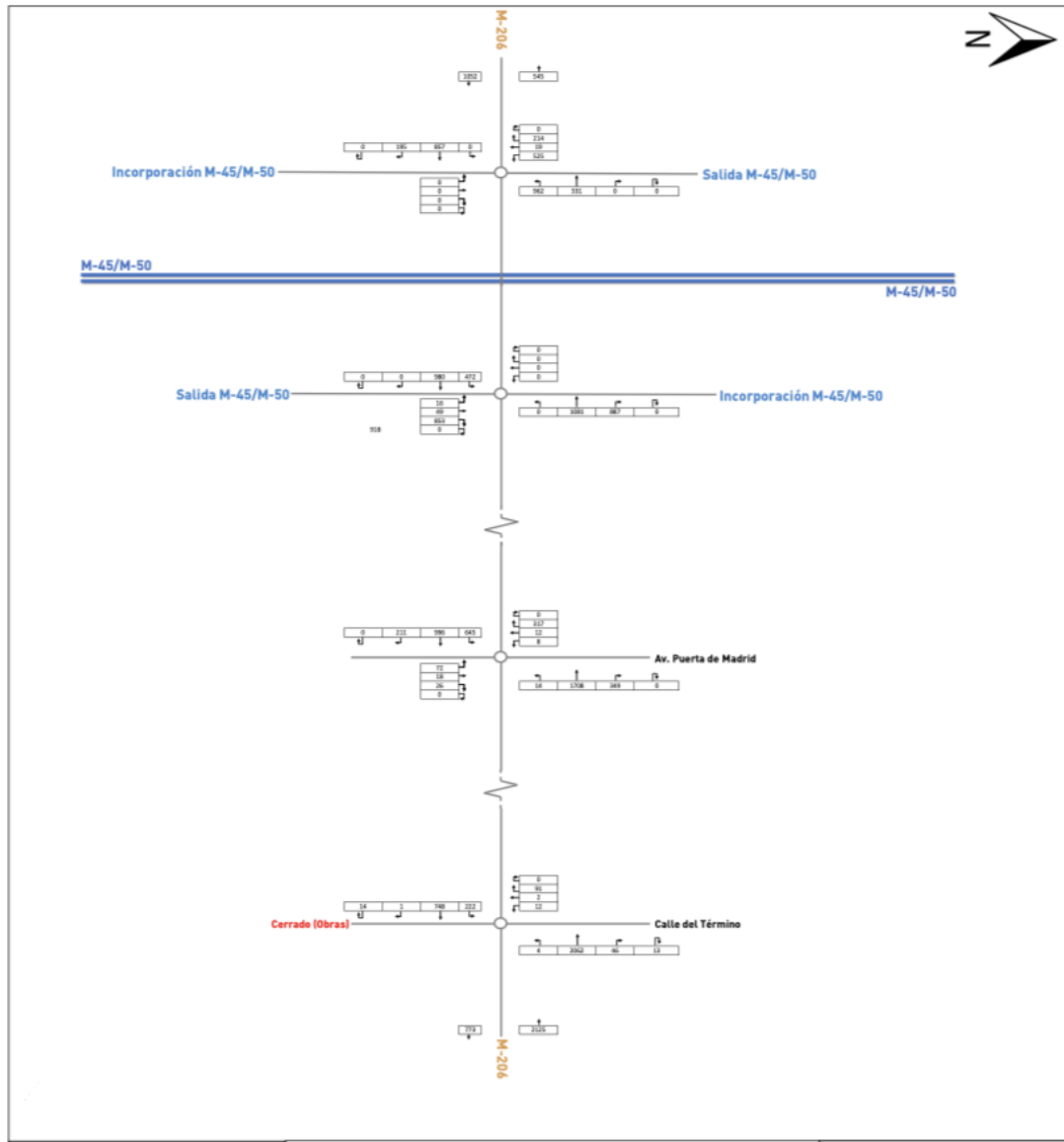
Imagen 19. Red de distribución del tráfico en hora punta AM (07:00–08:00).
